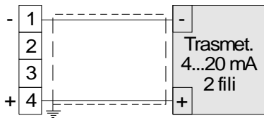
Fig. 4 Conexión 0/4-20 mA para transmisor pasivo usando fuente de alimentación auxiliar
