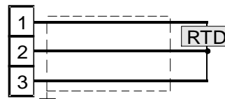
Fig. 4 Conexión RTD
